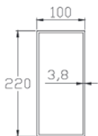
2 Профил рамка/колони
