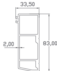
4 Преден профил
