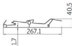
7 Ламелен профил
