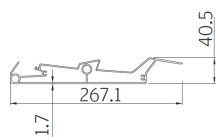
4 Ламелен профил
