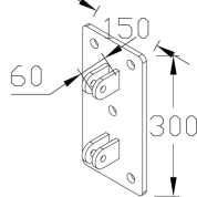
5 Стойка за захващане на стена
