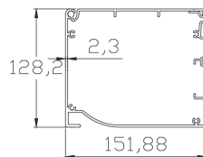
3 Кутия за мотор
