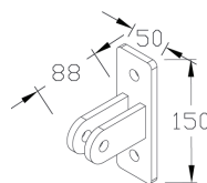
6 Предна стойка за захващане
