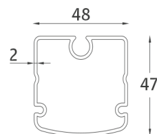
5 Поддържащ профил за плата
