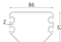
4 Изтеглящ профил за плата
