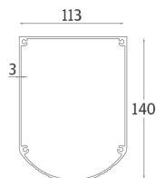
3 Профил колона
