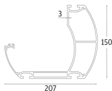
2 Водосточен профил
